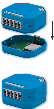
64-Serie met adapter EOA64
